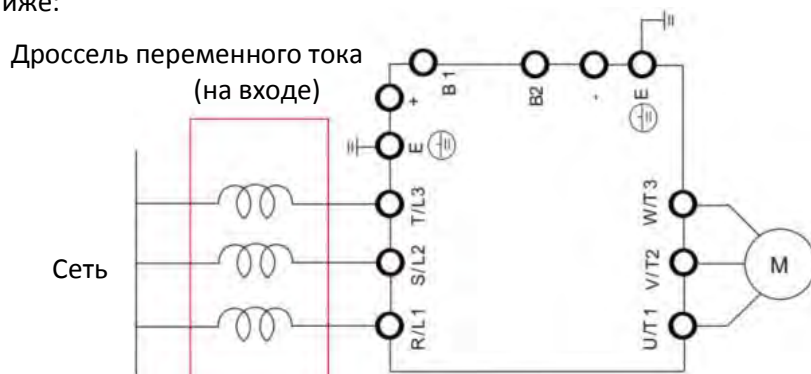
Подключение сетевого дросселя
