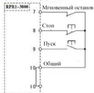
Трехпроводное управление
