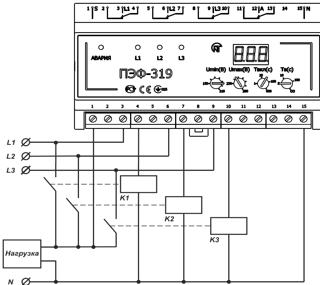
Рисунок 3 – Схема подключения ПЭФ-319 при величине нагрузки более 30 А с использованием магнитных пускателей
