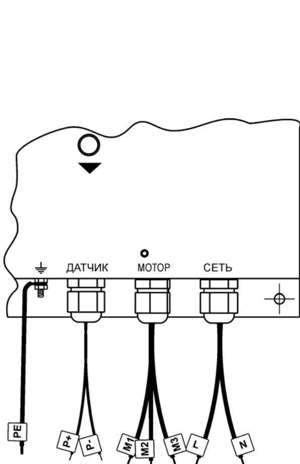
А – наименование проводов подключения
