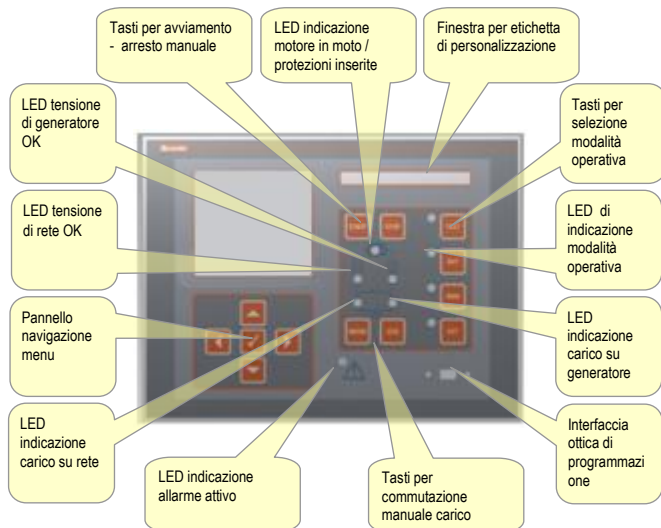
Pannello frontale RGK900
