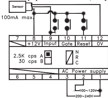
Счетчик с двумя уставками
