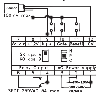
Счетчик с одной уставкой и непрерывного счета
