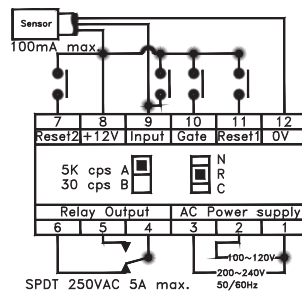
Счетчик с одной уставкой и непрерывного счета
