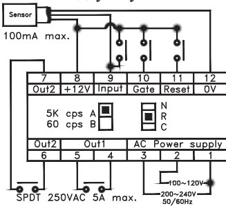
Счетчик с двумя уставками
