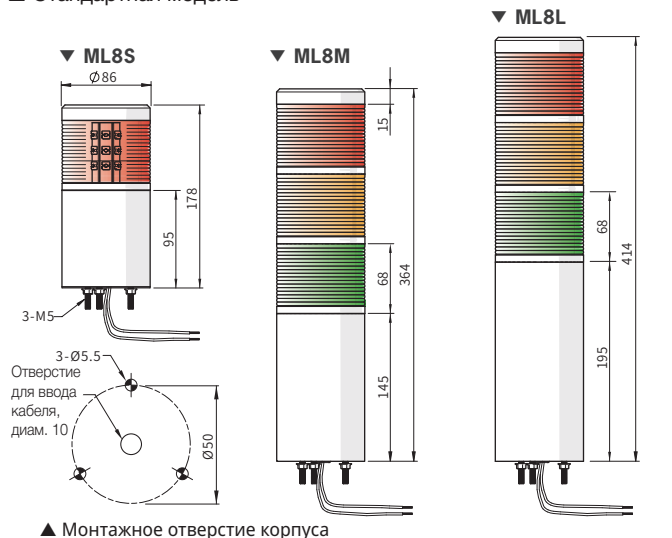
▲ Монтажное отверстие корпуса
