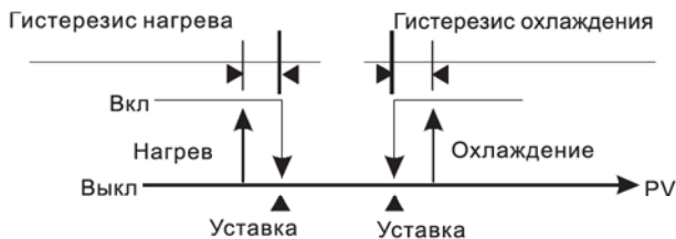
Рис1: Двухпозиционное регулирование для одного выхода
