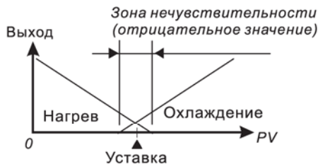
Рис 6: ПИД-регулирование. Двухконтурное управление с отрицательной зоной нечувствительности
