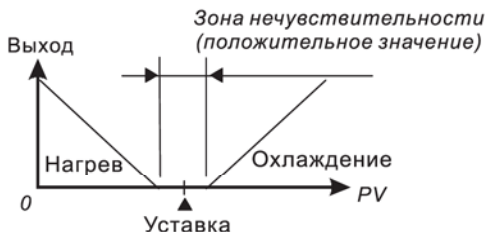
Рис 5: ПИД-регулирование. Двухконтурное управление с положительной зоной нечувствительности
