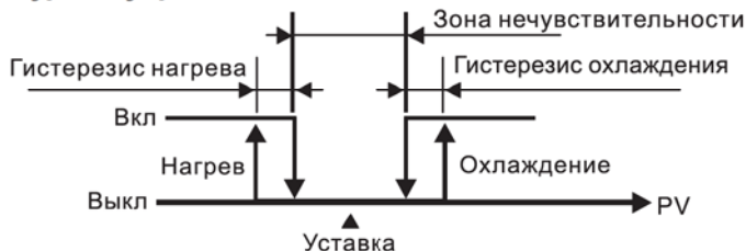
Рис4: Двухпозиционное регулирование при двухконтурном управлении
