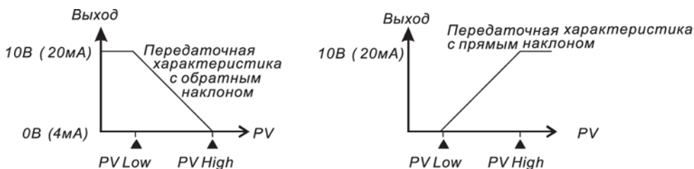
Рис 7: Пропорциональный выход
