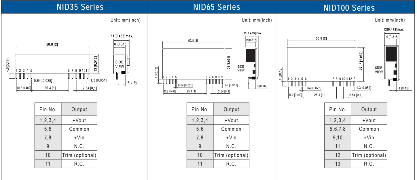
NID35 (2"x0.512"x0.433")
