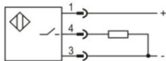
PNP NO
