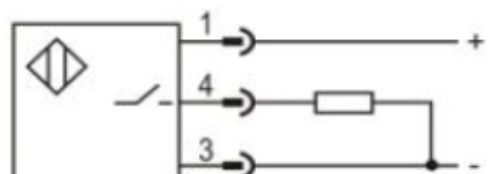
PNP NO
