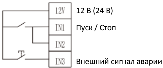
Двухпроводная система
