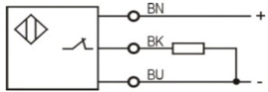
PNP NO
