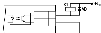
Рисунок 5.4 – Использование транзисторной оптопары для управления реле
