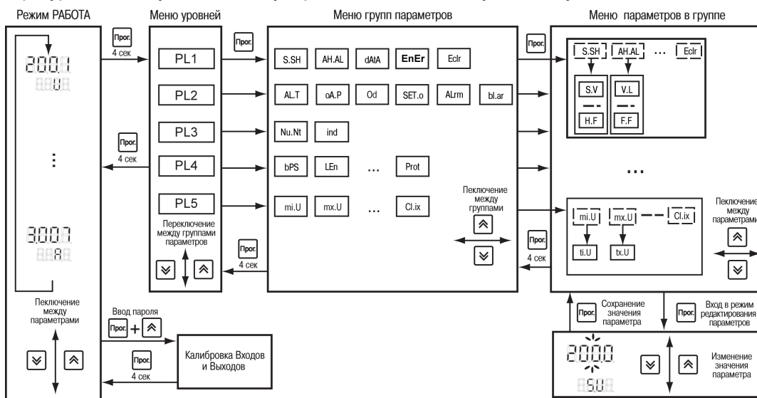
Рисунок 7.1 – Схема переходов по меню
