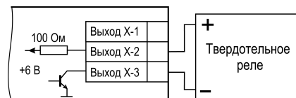
Рисунок 5.6 – Схема подключения к ВУ типа Т
