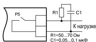
Рисунок 5.3 – Шунтирование контактов реле при работе с индивидуальными нагрузками
