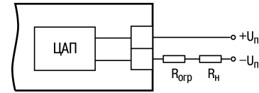
Рисунок 5.7 – Схема соединения ЦАП с нагрузкой
