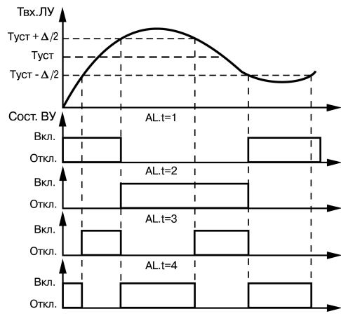
Рисунок 7.2 – Выходные характеристики компараторов
