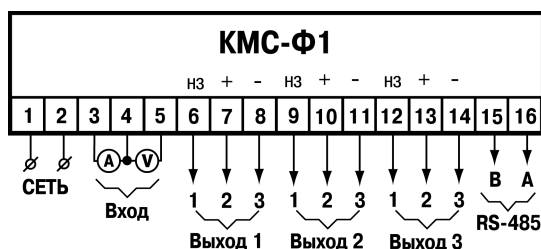
Рисунок 5.1 – Назначение клеммника
